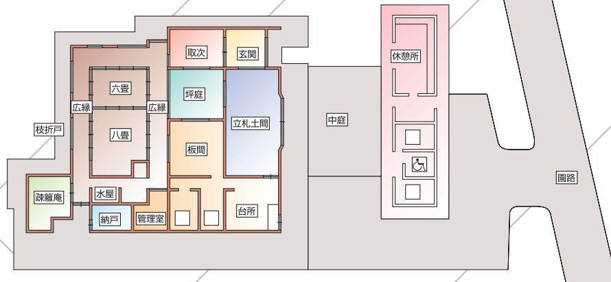
成蹊閣平面図
