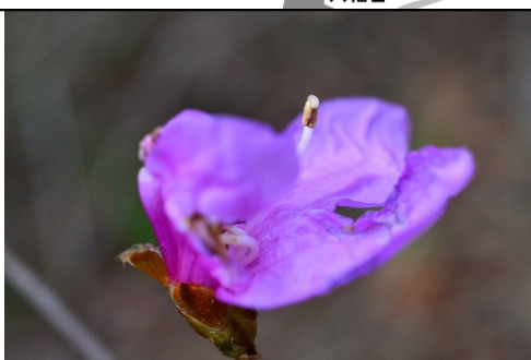
モチツツジの狂い咲き(左)とコバノミ ツバツツジの狂い咲き(右)
